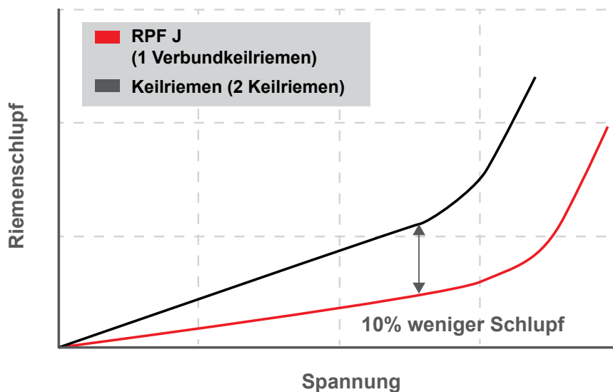
Riemenschlupf-Vergleich: RPF J vs. Keilriemen
